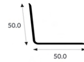
2° INTERNAL ANGLE
